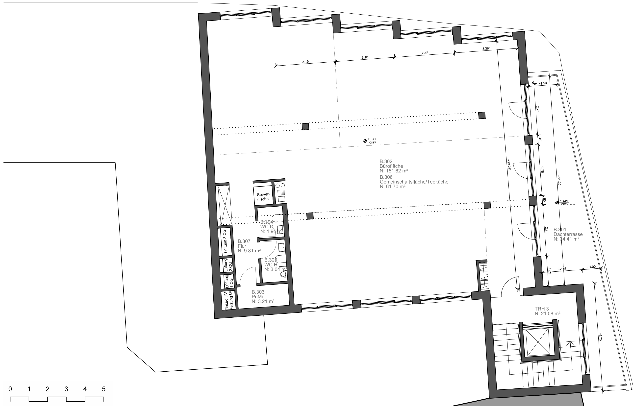
Grundriss BT B 3.OG | M 1:100
